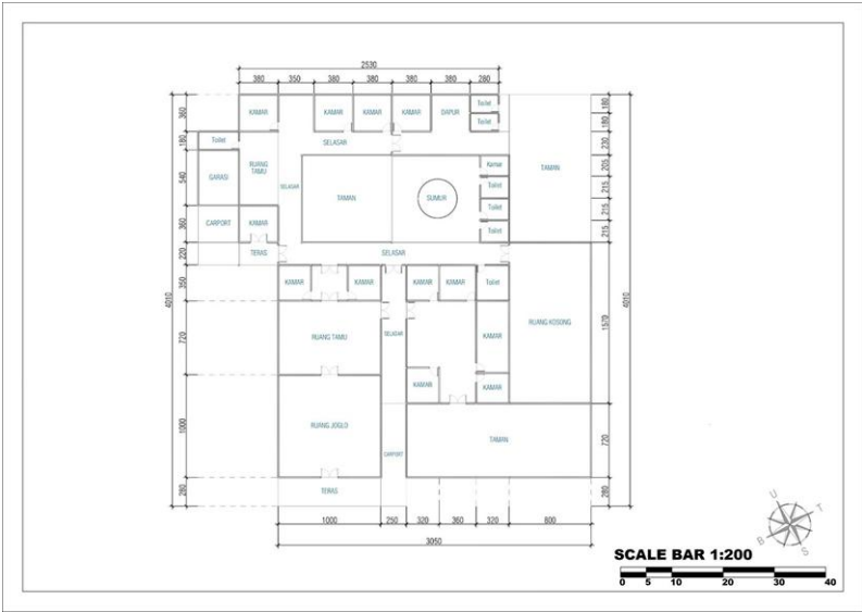
Gambar 2. Denah hubungan ruang dalam, ruang transisi, dan ruang luar Sumber: survei lapangan penulis, 2026
